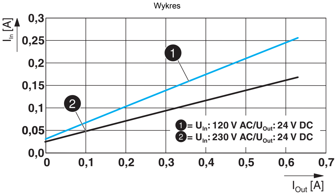
Prąd wejściowy/wyjściowy
