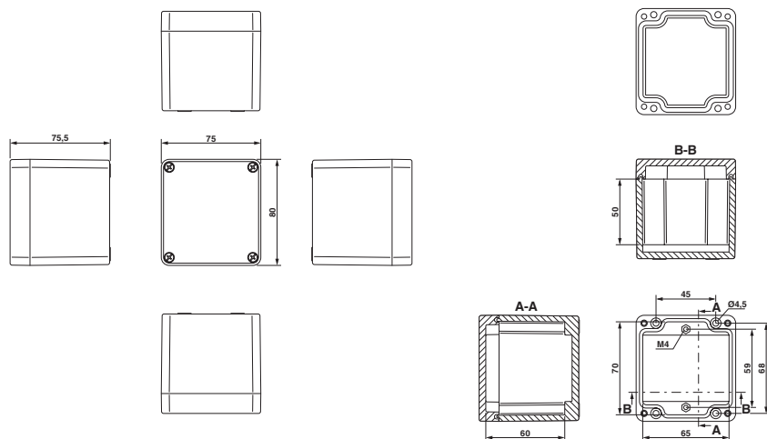
Rysunek wymiarowy
