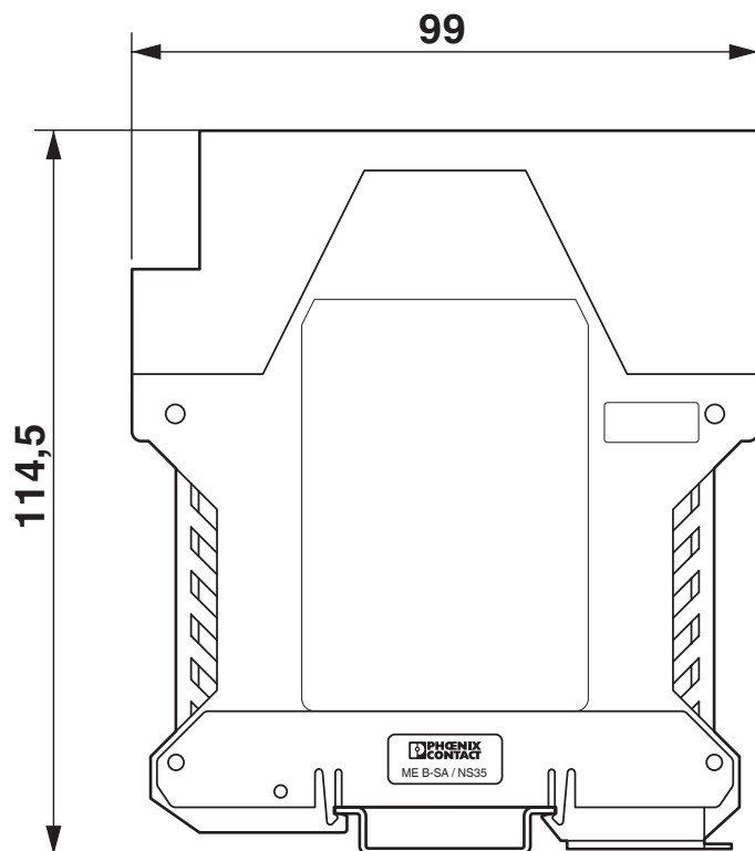
Rysunek wymiarowy
