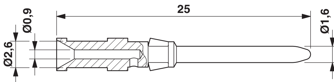
Rysunek wymiarowy
