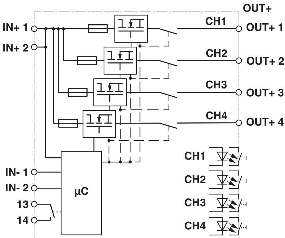
Schemat blokowy
