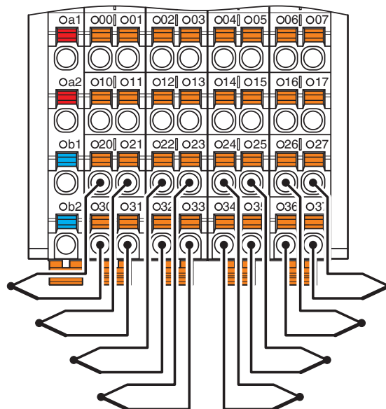
rysunek złączy
