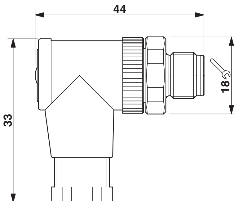
Rysunek wymiarowy
