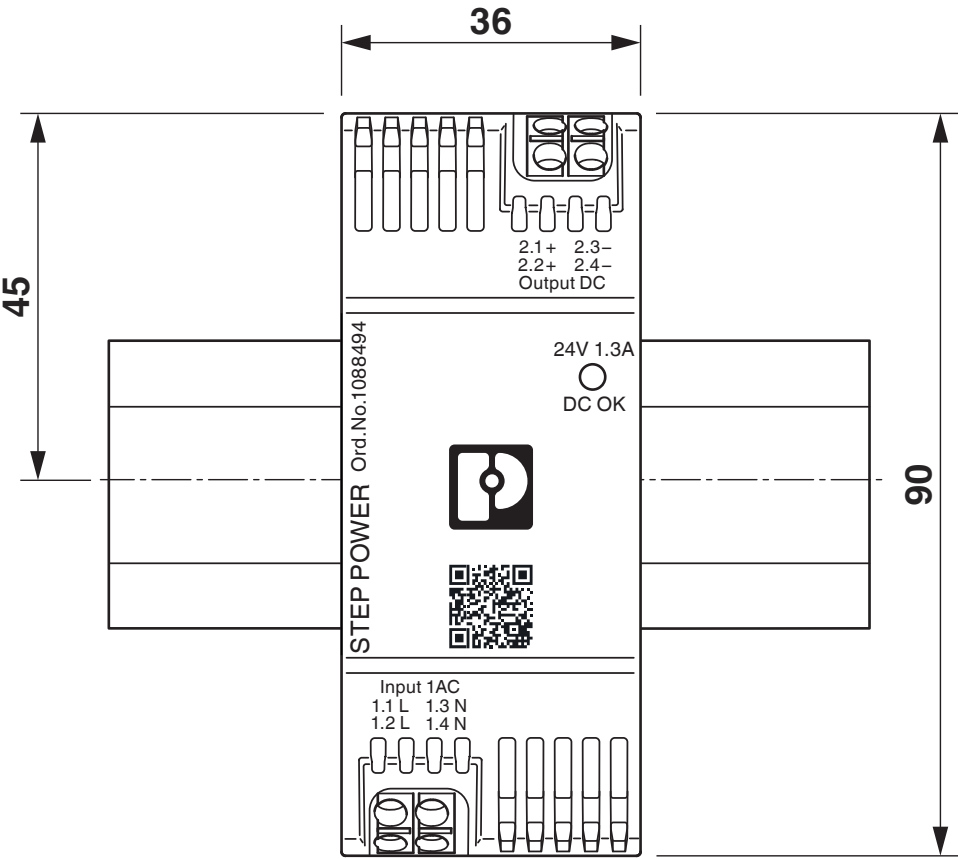
Rysunek wymiarowy
