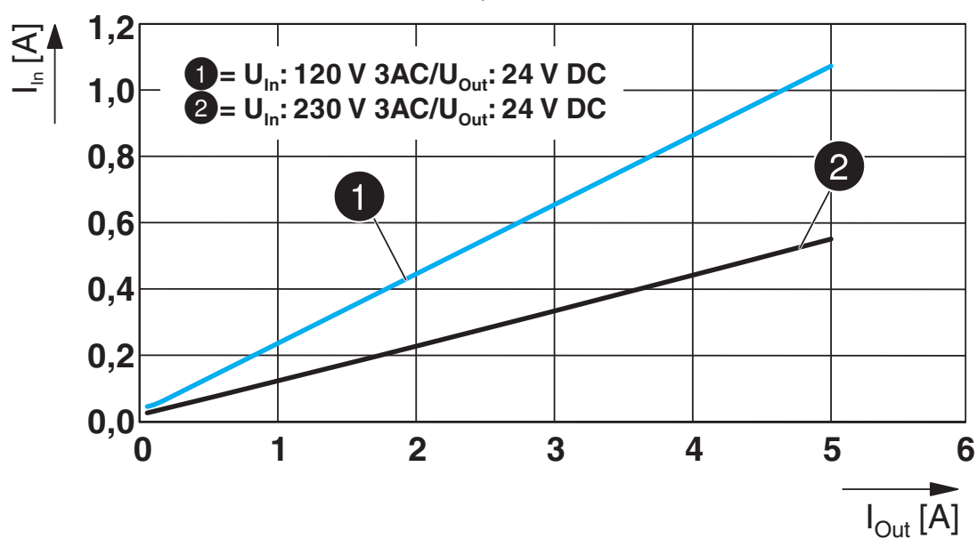
Prąd wejściowy/wyjściowy
