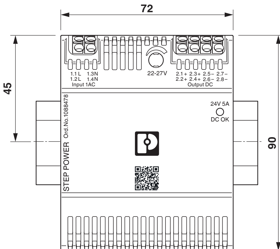
Rysunek wymiarowy
