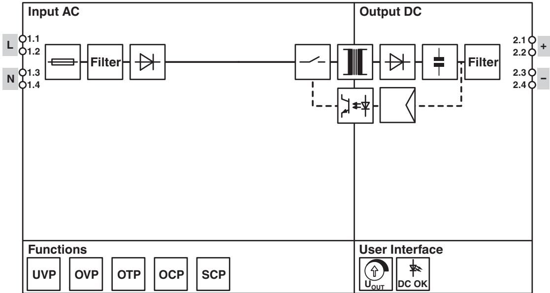
Schemat blokowy
