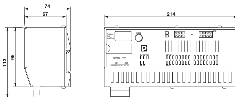
Rysunek wymiarowy
