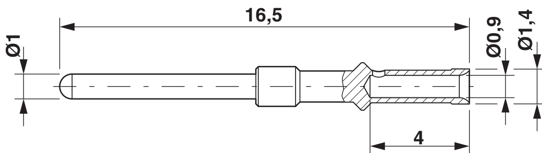
Rysunek wymiarowy
