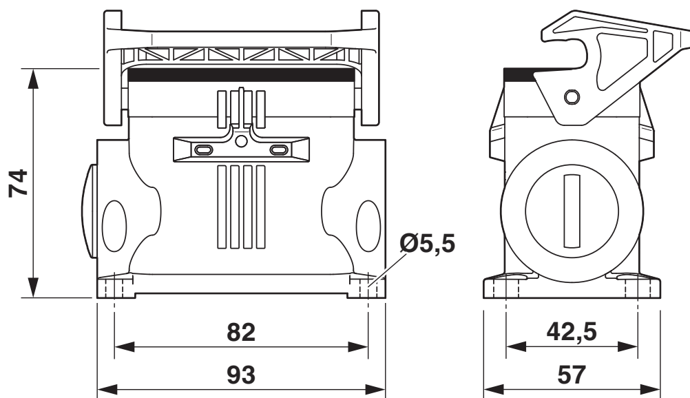
Rysunek wymiarowy
