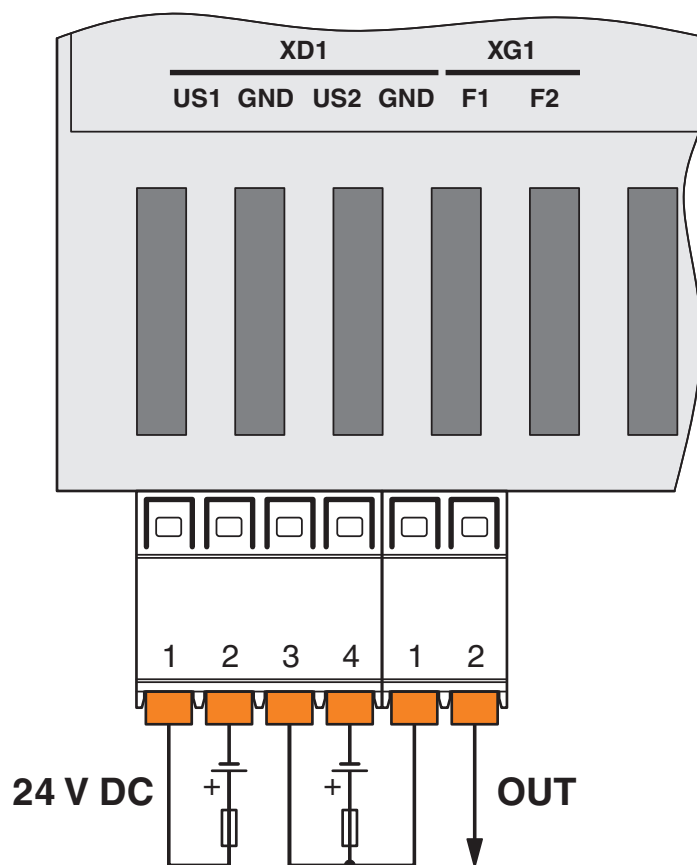
rysunek złączy
