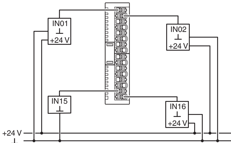
rysunek złączy
