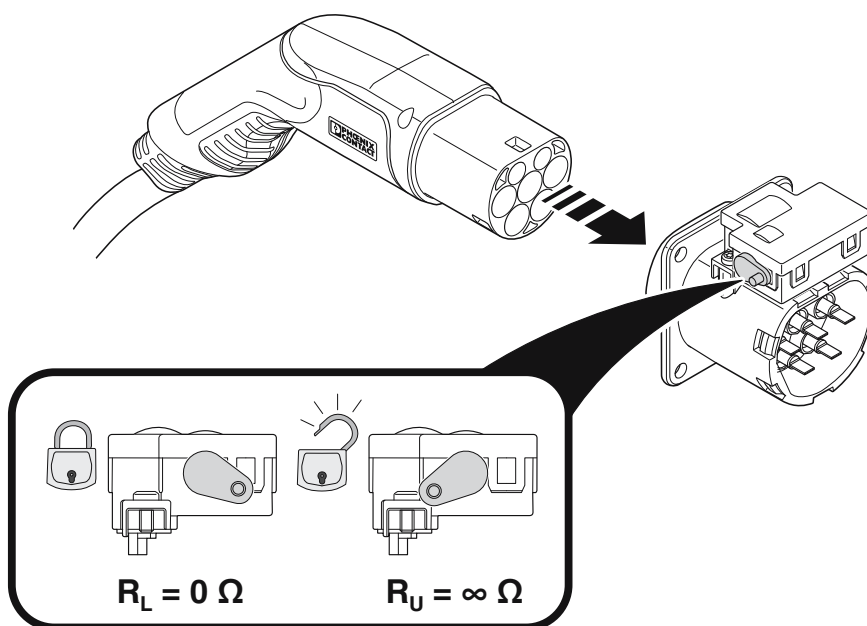
Rysunek schematyczny
