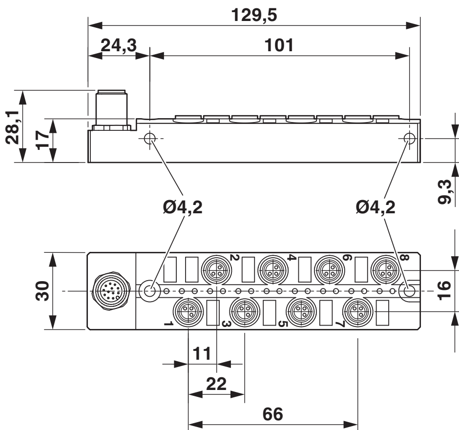
Rysunek wymiarowy
