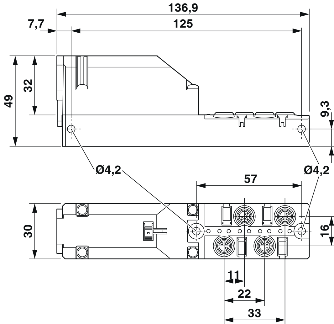
Rysunek wymiarowy
