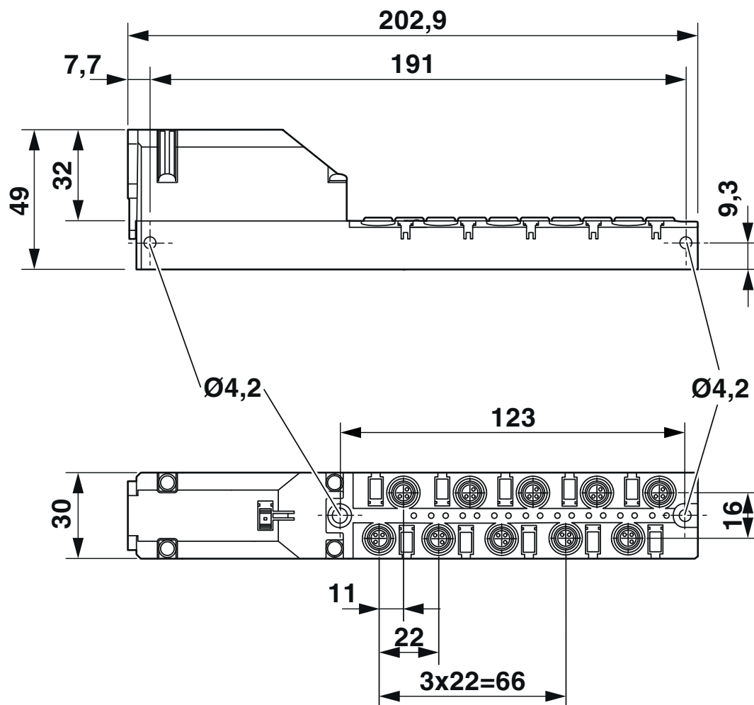
Rysunek wymiarowy
