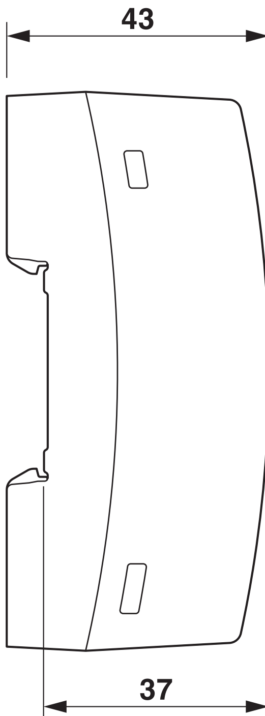
Rysunek wymiarowy
