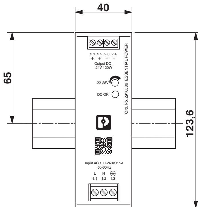
Rysunek wymiarowy
