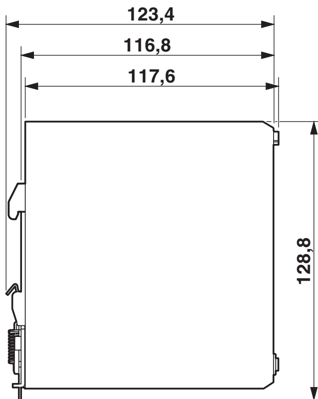
Rysunek wymiarowy
