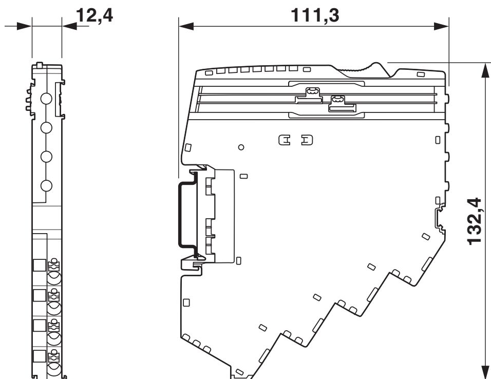
Rysunek wymiarowy
