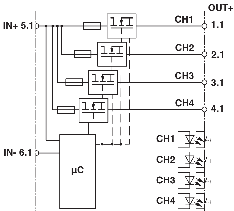
Schemat blokowy
