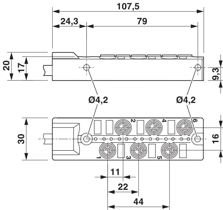
Rysunek wymiarowy
