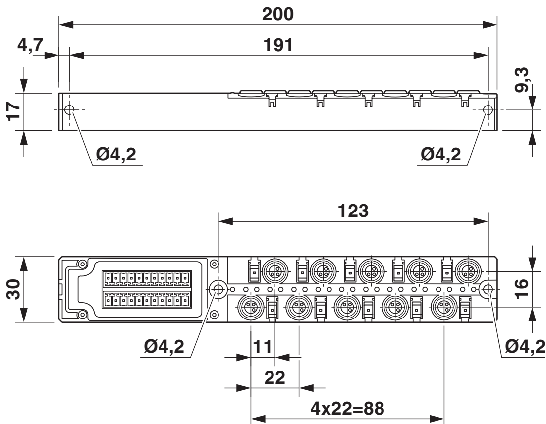
Rysunek wymiarowy
