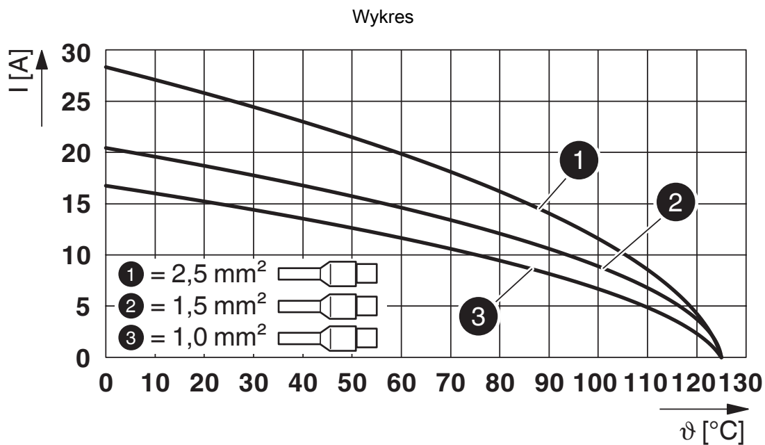
Wykres obniżenia parametrów znamionowych dla linii z tulejką
