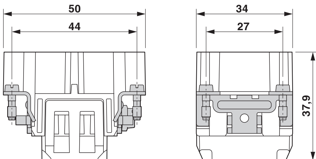
Wkładka styków męskich
