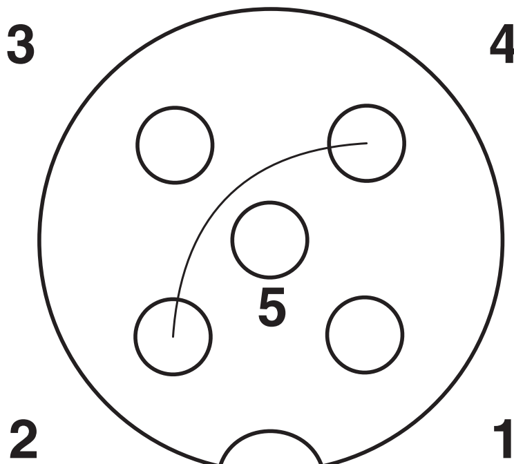
Układ styków, gniazdo M12, 3-bieg., zmostkowane, z PE, kod. A, od strony gniazda
