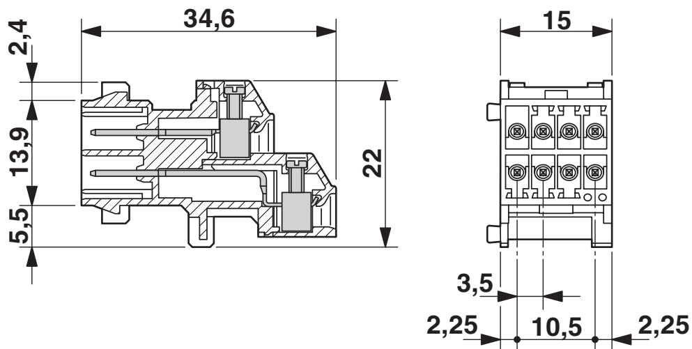
Rysunek wymiarowy
