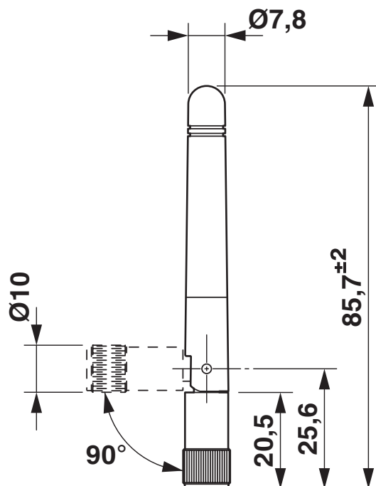
Rysunek wymiarowy
