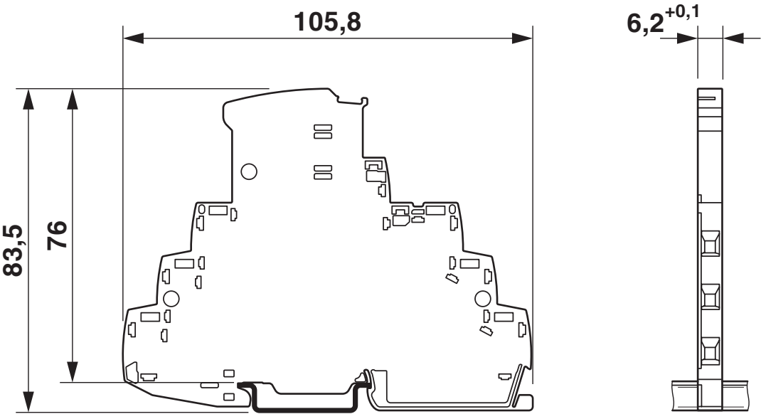
Rysunek wymiarowy
