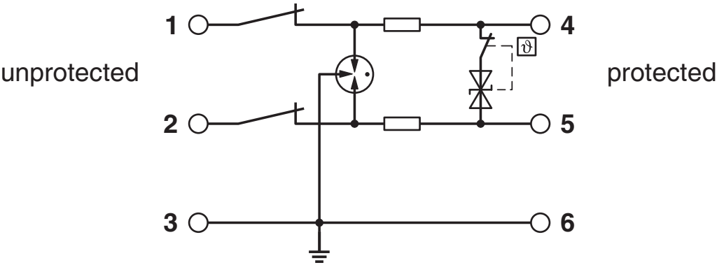
Schemat
