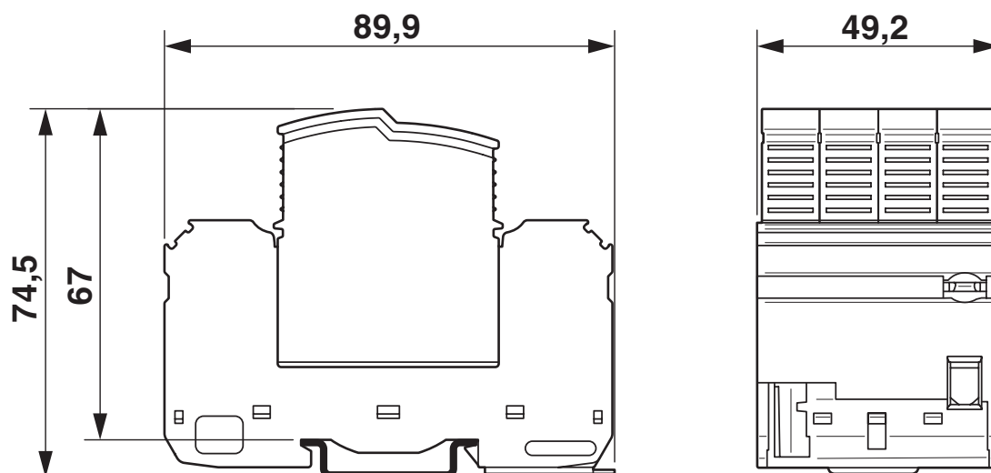
Rysunek wymiarowy
