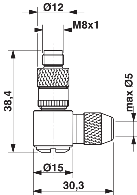
Rysunek wymiarowy
