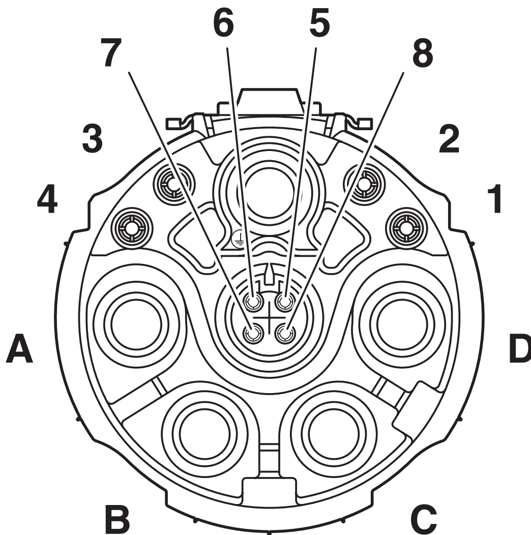
Układ styków złącza żeńskiego sygnałowego, kodowanie 1
