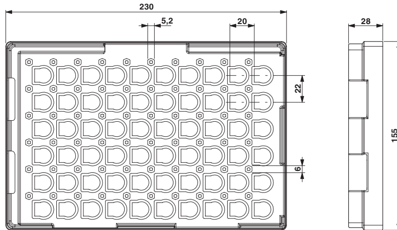
Rysunek wymiarowy
