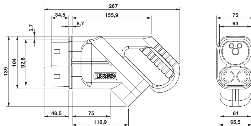
Rysunek wymiarowy
