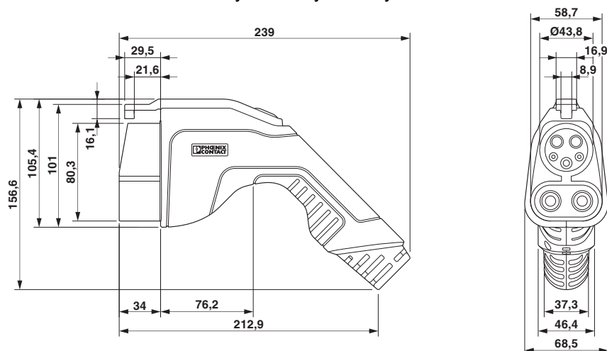
Rysunek wymiarowy
