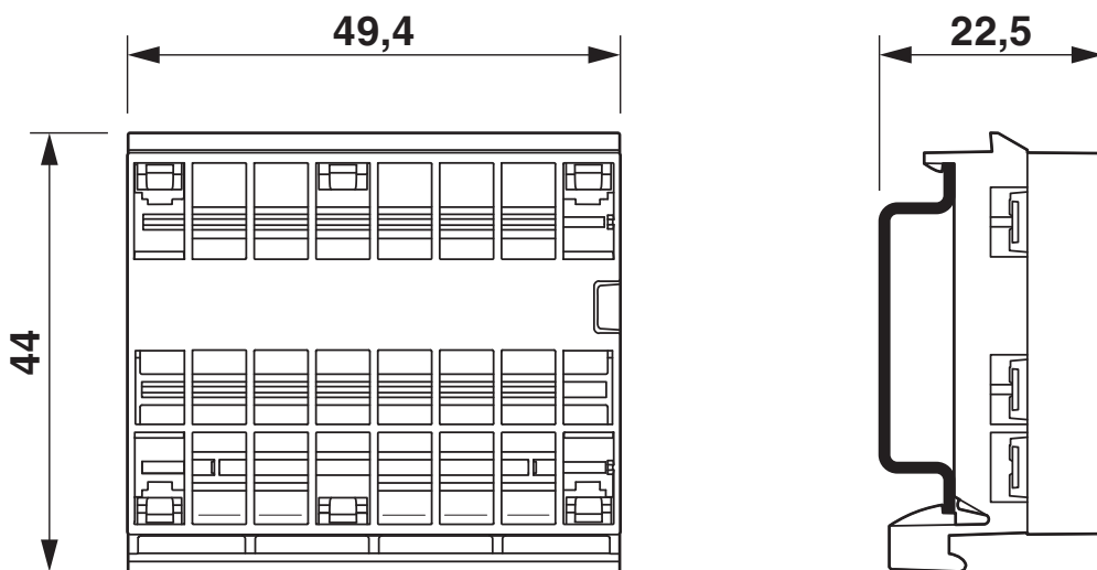
Rysunek wymiarowy
