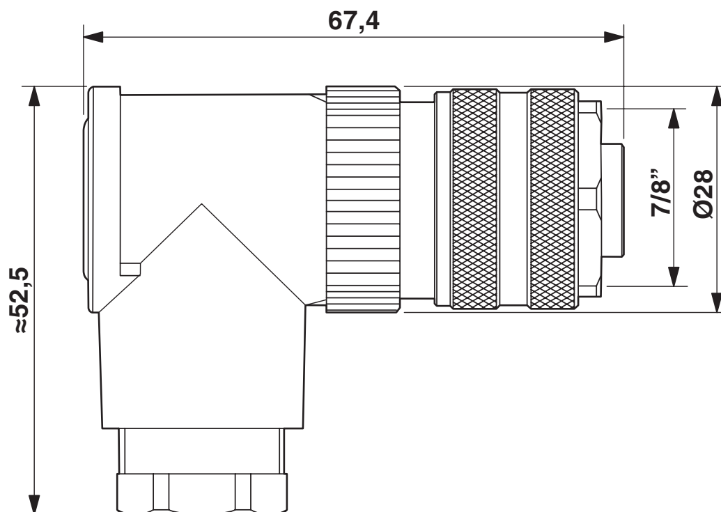
Rysunek wymiarowy
