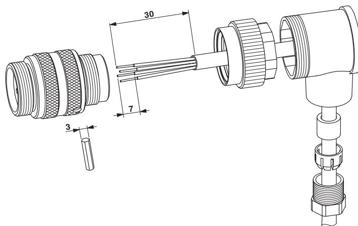
rysunek funkcyjny
