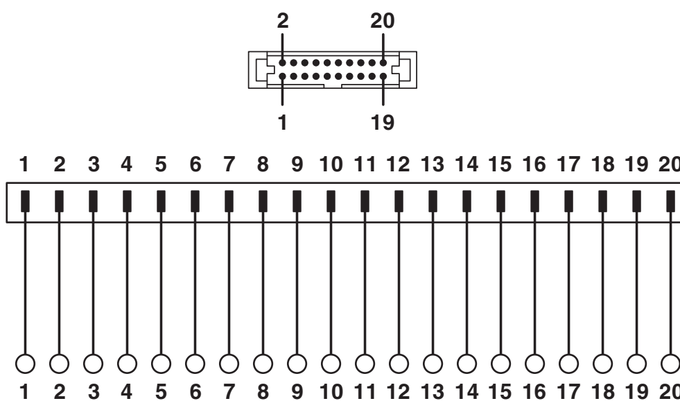
Schemat
