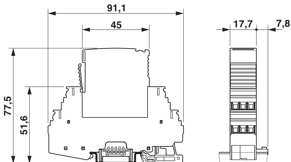
Rysunek wymiarowy
