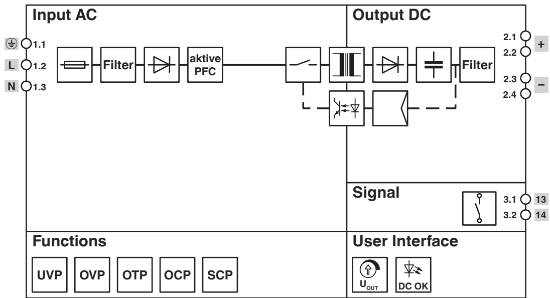
Schemat blokowy
