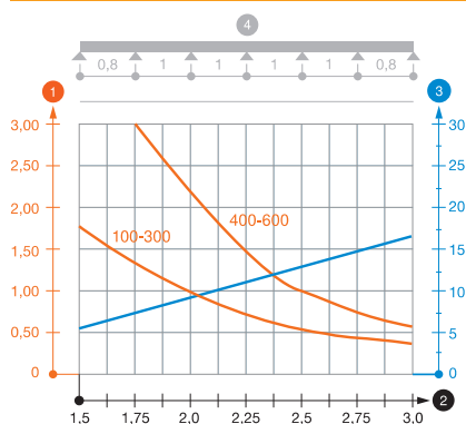
Wykres obciążenia korytka kablowego DKS 60 VA
