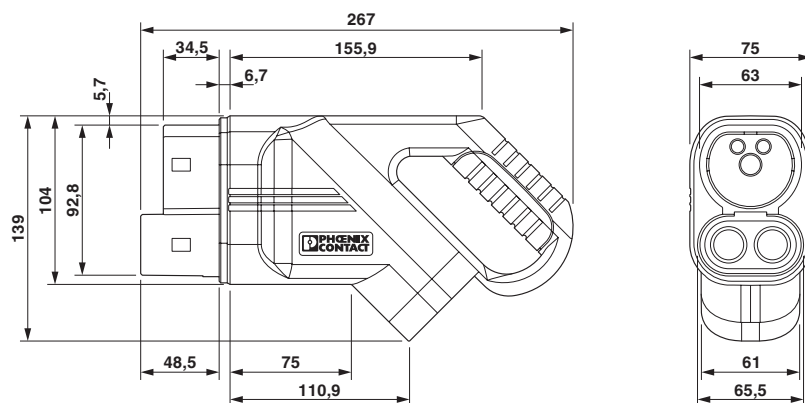
Rysunek wymiarowy
