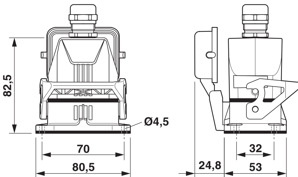
Rysunek wymiarowy
