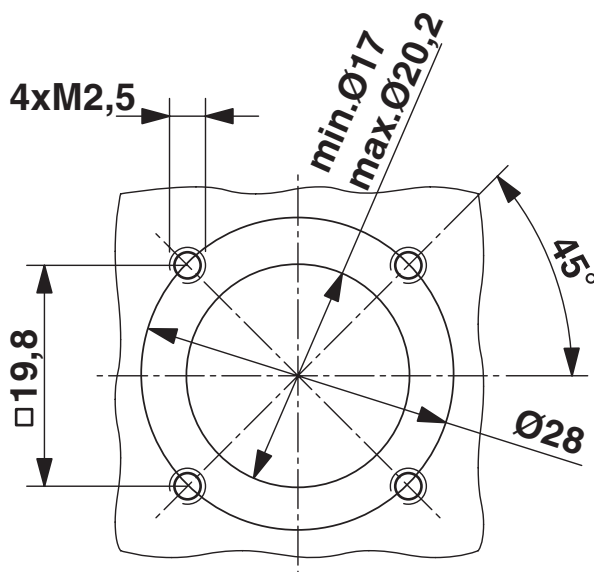
Rysunek wymiarowy
