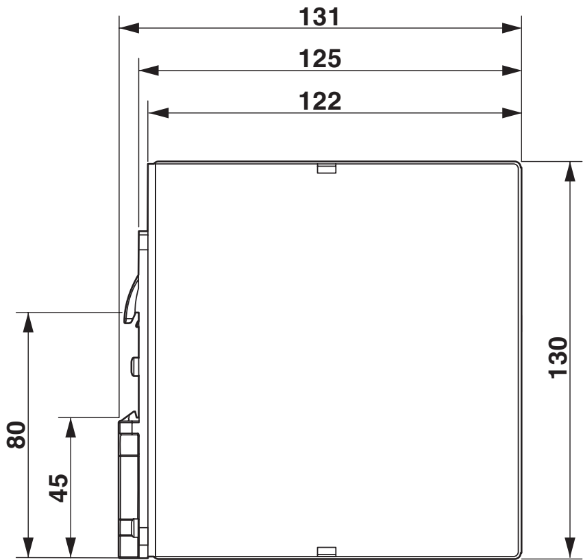
Rysunek wymiarowy
