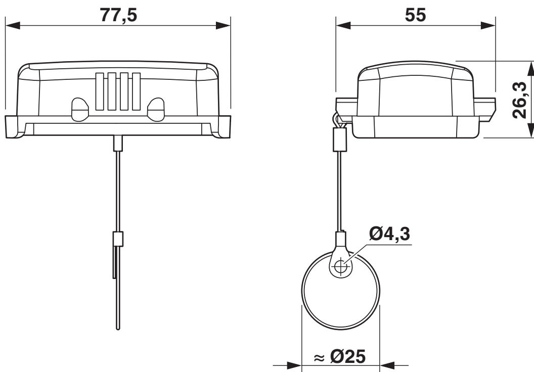
Rysunek wymiarowy
