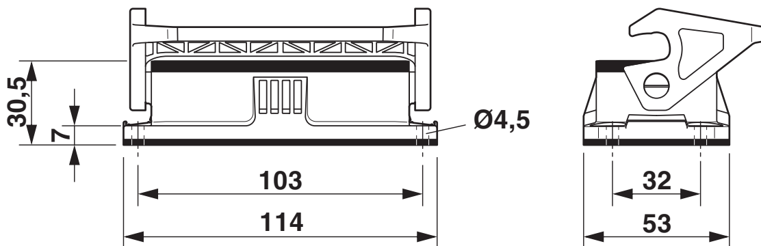
Rysunek wymiarowy
