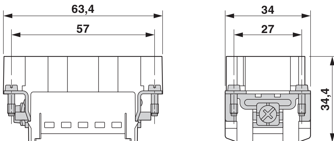
Rysunek wymiarowy
